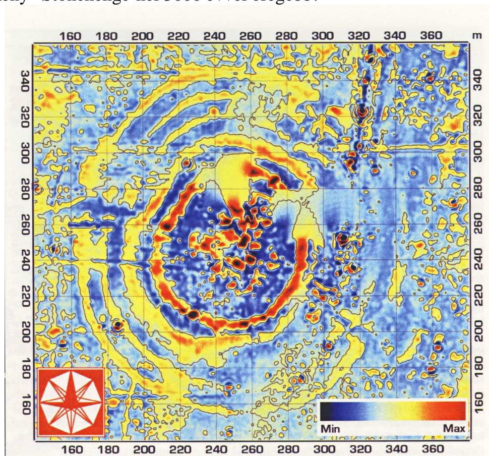
Polgár-Csőszhalom 7300 éves, ötszörös körárok-rendszerének mágneses térképe.
